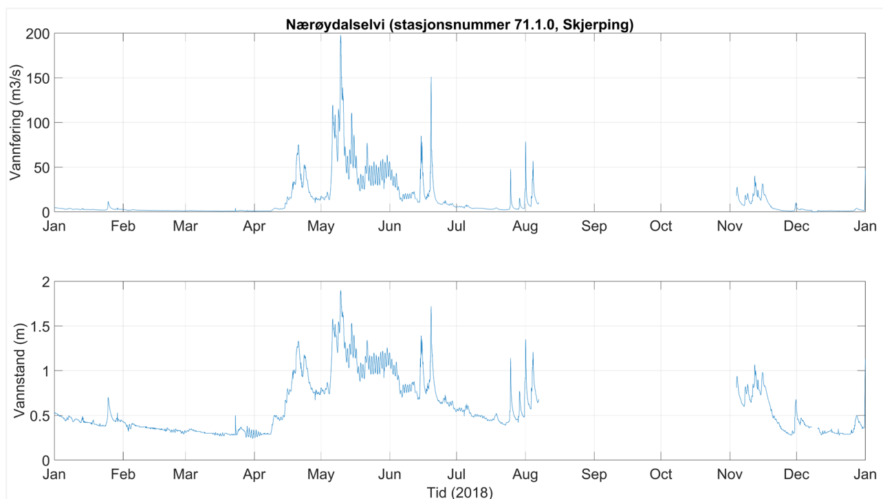
Figur 28. Vannføring og vannstand gjennom 2018 for Nærøydalselvi. Data hentet fra sildre.nve.no .
