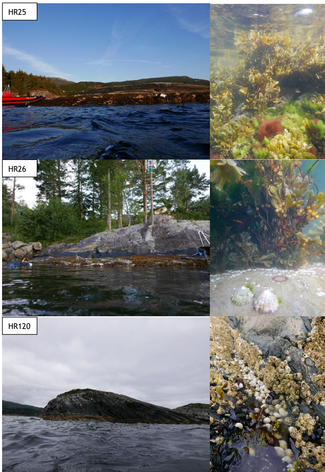
Figur 5. Bilder fra hardbunnstasjonene HR25, HR26 og HR120 i DP Nordsjøen Nord. Oversiktsbilde av stasjonene er gitt i venstre kolonne og bilde fra stasjonenes fjæresone er gitt i høyre kolonne (Foto: NIVA)
