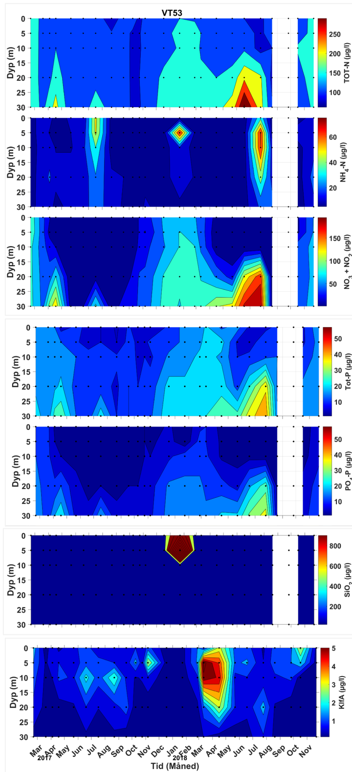
Figur 26. Næringssalter og klorofyll a som funksjon av tid og dyp for stasjon VT53 Tveiteneset i perioden 2017 til 2018. For september 2018 mangler det næringssalter for alle dyp. Dette er rapportert som avvik tidligere.
