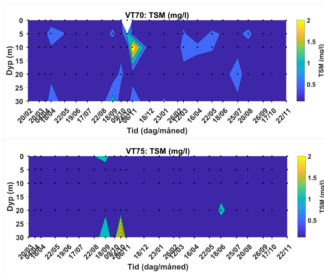
Figur 29. Variasjon over tid og dyp for TSM-konsentrasjoner VT70 Bjørnafjorden og VT75 Fusafjorden 2017-2018.
