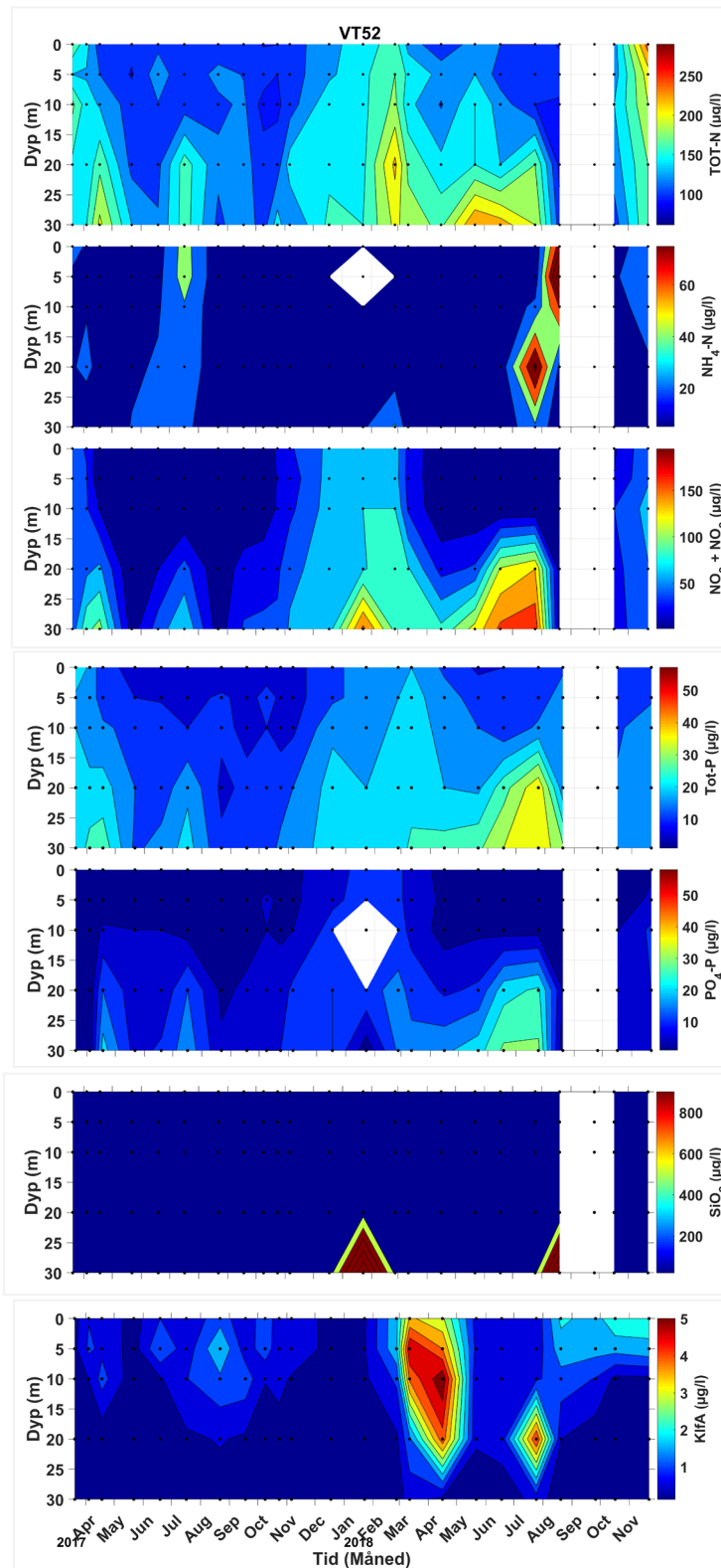
Figur 24. Næringssalter og klorofyll a som funksjon av tid og dyp for stasjon VT52 Kvinnheradsfjorden i perioden 2017 til 2018. For september 2018 mangler det næringssalter for alle dyp. Dette er rapportert inn.
