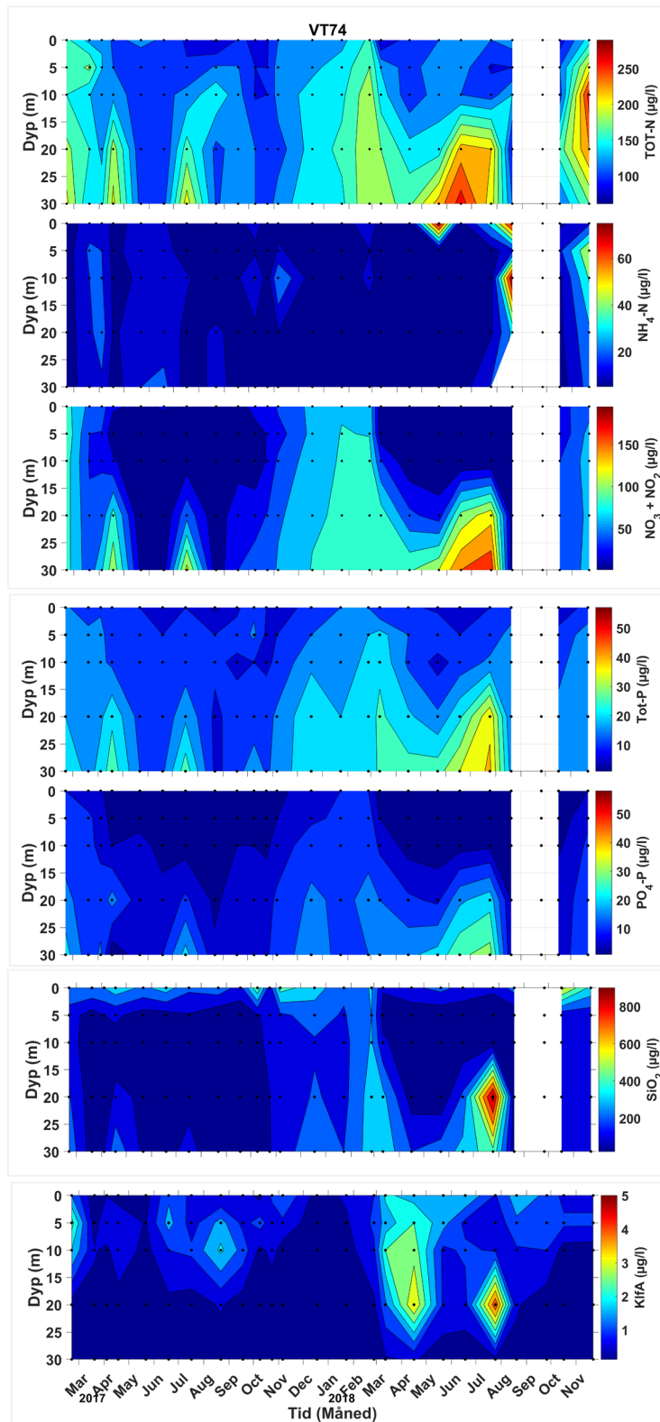
Figur 25. Næringssalter og klorofyll a som funksjon av tid og dyp for stasjon VT74 Maurangsfjorden i perioden 2017 til 2018. For september 2018 mangler det næringssalter for alle dyp. Dette er rapportert inn. \text{NH}_4\text{-N} fra 30 m i august 2019 er satt som NaN ettersom verdien er mistenkelig høy.
