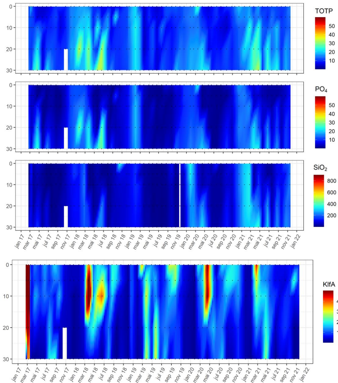
Figur 55. Næringssalter og klorofyll a som funksjon av tid og dyp for stasjon VT8 i perioden 2017 til 2021. Data fra 2017 til februar 2021 er hentet fra Vannmiljø. De svarte prikkene er prøvetidspunkt og prøvetakningsdyp.
