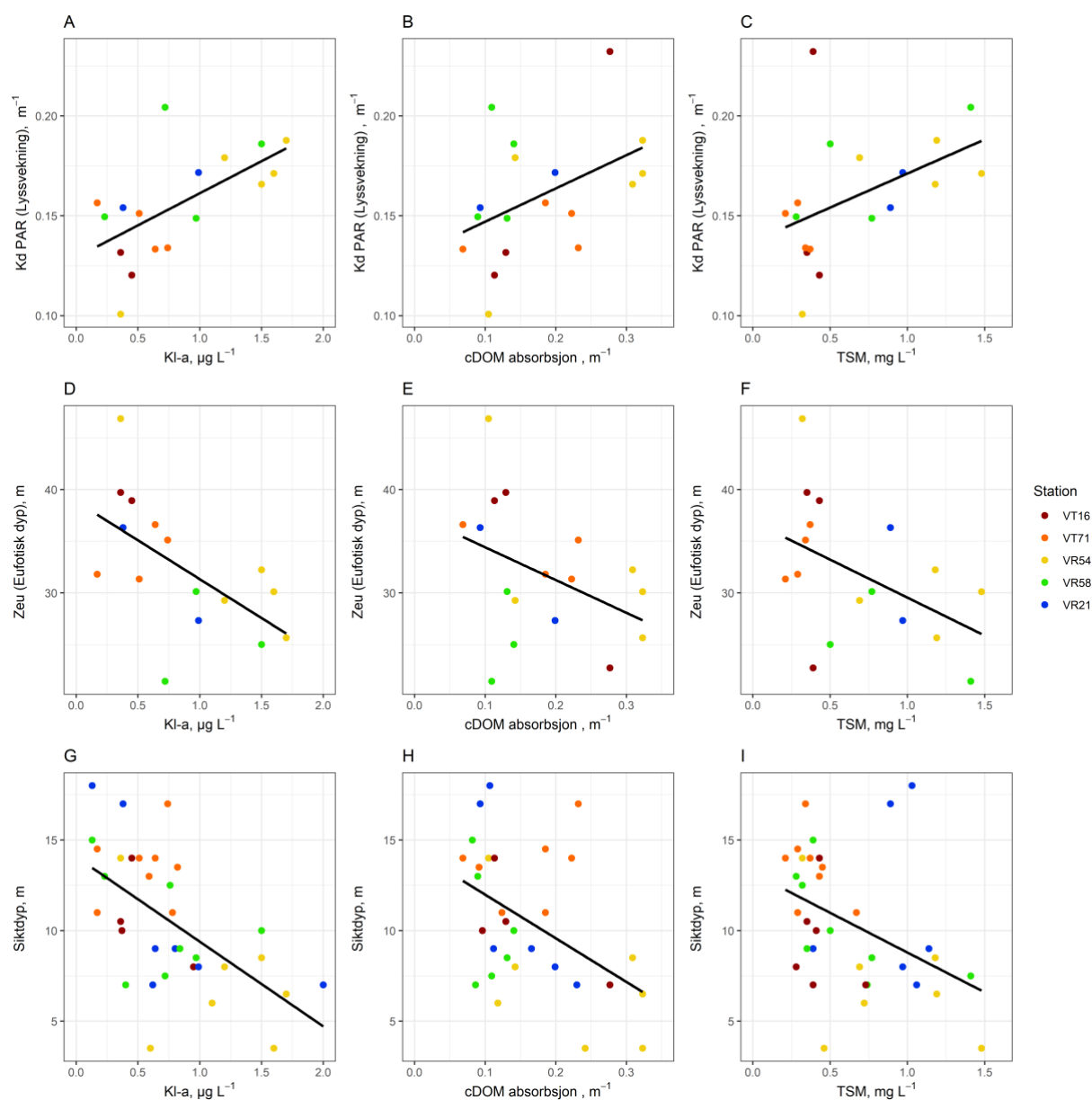
Figur 77. K_d PAR, lyssvekningskoeffisienten ( m^{-1} ), Zeu, eufotisk dyp (m) og siktdyp (m) i relasjon til andre klimaparameterer; Klorofyll a (A, D og G), cDOM absorpsjon (B, E og H) og TSM (C, F og I). Farger indikerer de ulike stasjonene.
