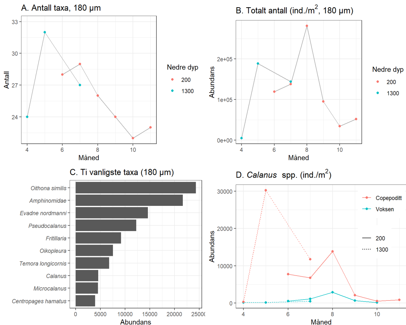
Figur 80. Sesongvariasjon i dyreplanktonsamfunnet (180 µm-fraksjon). A: Antall taxa observert i prøvene per måned, skilt på prøver fra de øvre 200 m og fra hele vannsøylen (1300 m). B: Beregnet totalantall dyreplankton i vannsøylen per måned på tvers av arter og stadier, skilt på prøver fra de øvre 200 m og fra hele vannsøylen (1300 m). C: De ti mest tallrike taxa observert gjennom året (gjennomsnitt for alle måneder). D: Antall av de ulike stadiene av Calanus spp. per måned, skilt på prøver fra de øvre 200 m og fra hele vannsøylen (1300 m) (stasjon VT16 Kyrkjebø).
