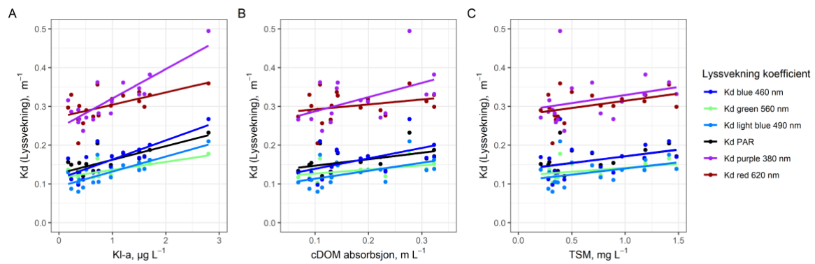
Figur 78. Lyssvekningskoeffisienter ( K_d m^{-1} ) for ulike deler av spektra og PAR fra stasjon VR54 (enkeltmålinger mai- september 2021) i relasjon til andre klimaparameterer; Klorofyll a (A), CDOM absorpsjon (B) og TSM (C). Farger indikerer de ulike bølgelengdene; sort: PAR 400-700 nm, fiolett: 380nm, mørk blå: 460nm, lys blå: 490 nm, grønn: 540 nm og rød: 620 nm.
