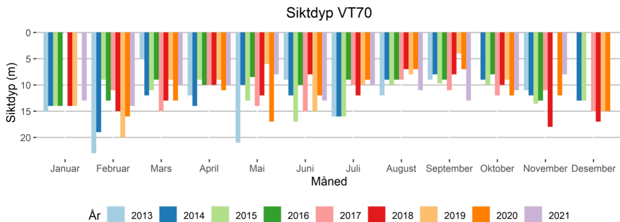
Figur 65. Siktdyp i meter for stasjonen VT70 Bjørnafjorden fra 2013 til 2021.
