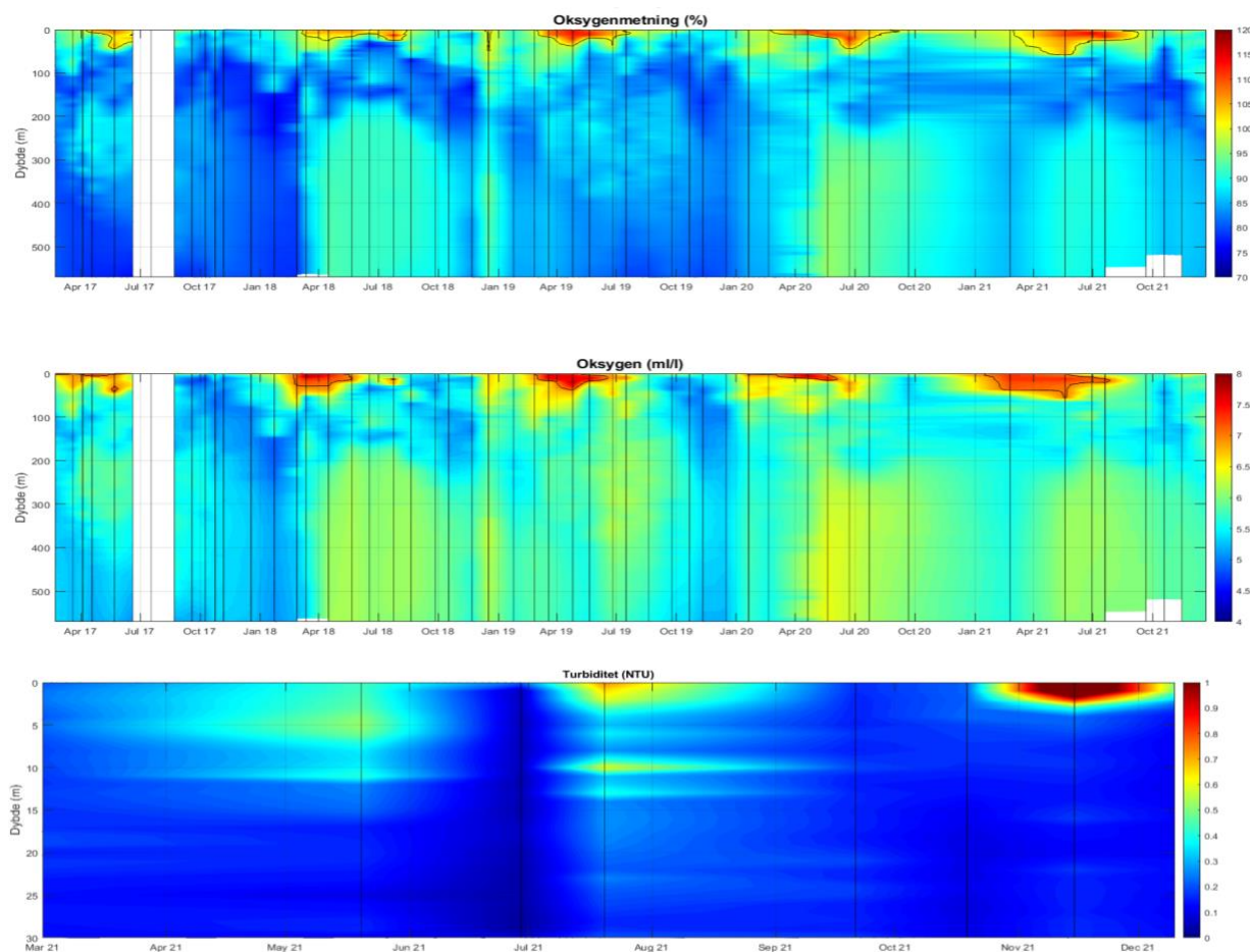
Figur 49. Data fra CTD-målinger på stasjon VT70 Bjørnafjorden. Øverst vises konturplott av saltholdighet med en fargeskala fra 25 til 35. Under saltholdighetsplottet vises konturplott av temperatur med en fargeskala fra 2 til 18 °C. Under temperaturplottet vises et konturplott av oksygenmetningen med en fargeskala fra 70 til 120%. Videre vises oksygenkonsentrasjonen med en fargeskala fra 4 til 8 ml/L. Nederst vises turbiditet fra 2021 for de øvre 30 meterne med en fargeskala fra 0 til 1. Sorte streker indikerer dato for når observasjonene ble gjort. Hvite felt indikerer manglende data.
