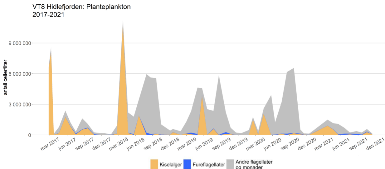
Figur 91. VT8 Hidlefjorden. Fordelingen av planteplankton på grupper fra 2017 til 2021 på 5 m dyp. Gruppen andre flagellater og monader består av kiselflagellater, svelgflagellater, grønnalger, olivengrønnalger, øyealger, svepeflagellater, kalkflagellater, ubestemte monader og ubestemte flagellater.
