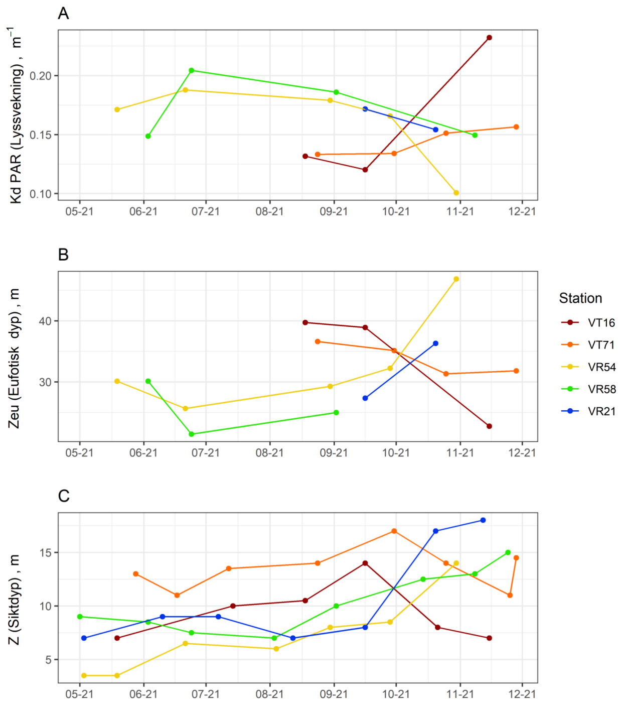
Figur 75. Plot av lys mellom mai til november 2021 per stasjon; (A) Lyssvekningskoeffisienten til nedoverrettet 1 % diffust lys integrert for PAR (Photosynthetically Active Radiation, K_d\_PAR\ m^{-1} ), (B) Eufotisk dyp (Zeu, m) og (C) Siktdyp (m). Farger indikerer de ulike stasjonene fra syd til nord.
