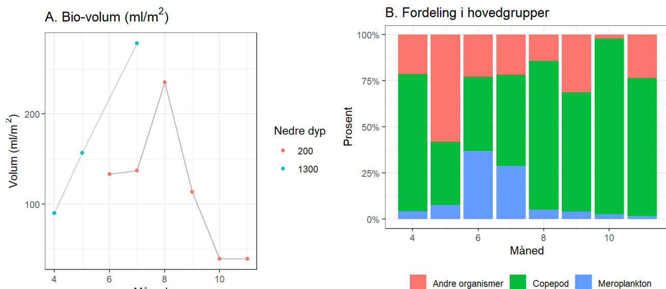
Figur 79. A: Sesongvariasjon i bio-volum (det totale volumet av biologisk materiale i prøven). B: Fordeling av dyreplankton i hovedgrupper per måned (abundans) (stasjon VT16 Kyrkjebø).
