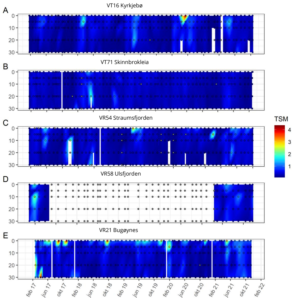
Figur 71. 5-års tidsserie (2017-2021 av totalt suspendert materiale (TSM) i 0-30 m dyp for klimastasjonene VT16 Kyrkjebø (A), VT71 Skinnbrokleia (B), VR54 Straumsfjorden (C), VR58 Ulsfjorden (D), og VR21 Bugøynes (E).
