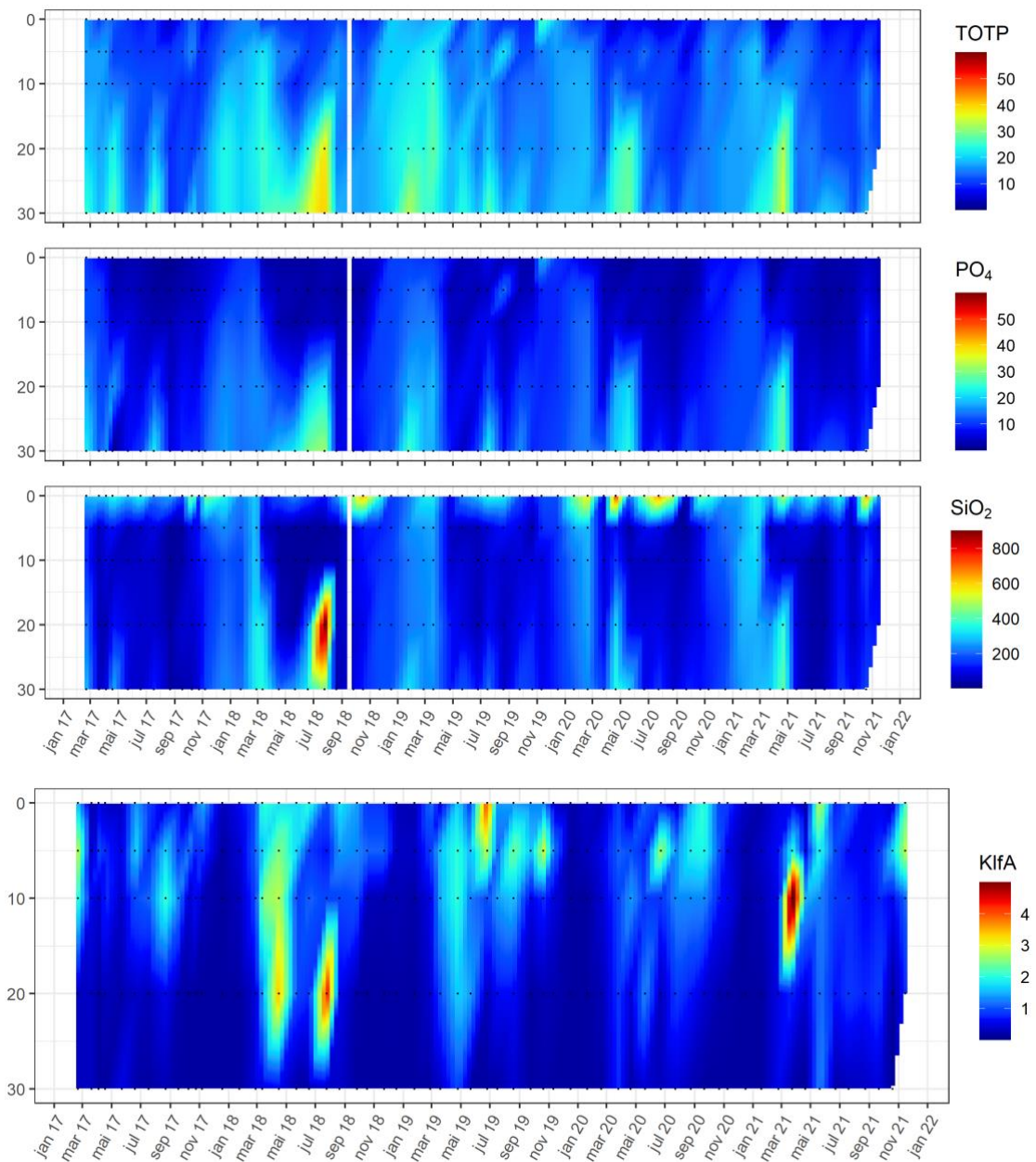
Figur 61. Næringssalter og klorofyll a som funksjon av tid og dyp for stasjon VT74 Maurangsfjorden i perioden 2017 til 2021. For september 2018 mangler det næringssalter for alle dyp, og dette er rapport tidligere. Hvite felter er data som er fjernet under kvalitetskontroll. De svarte sirklene er prøvetidspunkt og prøvetakningsdyp.
