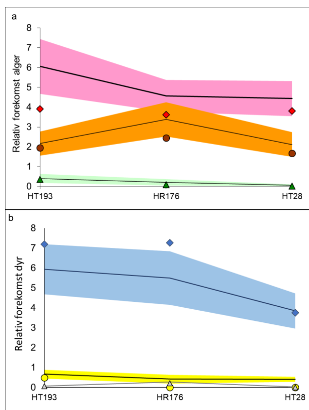
Figur 9. Relativ forekomst av a) makroalger og b) bentiske dyr på hardbunn summert over dypintervallet 4 til 22 m. Makroalgene er delt opp i rødalger (◇ rosa), brunalger (● oransje) og grønnalger (Δ grønn). Dyrene er vist for vannfiltrerende dyr (◇ blå), rovdyr (● gul) og plantebeitere (Δ grå). Punktene er årets registreringer, linje er snittet fra 1990-2020, fargede områder er snitt +/- stdev. Relativ forekomst er beregnet som summen av forekomsten (over dypintervallet 4 til 22 m) pr. stasjon, pr. år / 100.
