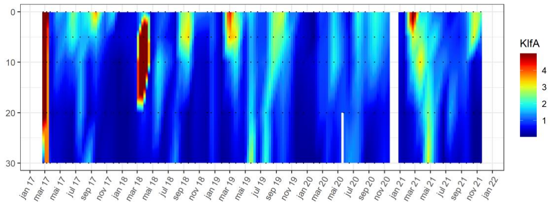
Figur 56. Næringssalter og klorofyll a som funksjon av tid og dyp for stasjon VT83 i perioden 2017 til 2021. Data fra 2017 til februar 2021 er hentet fra Vannmiljø. De svarte prikkene er prøvetidspunkt og prøvetakningsdyp
