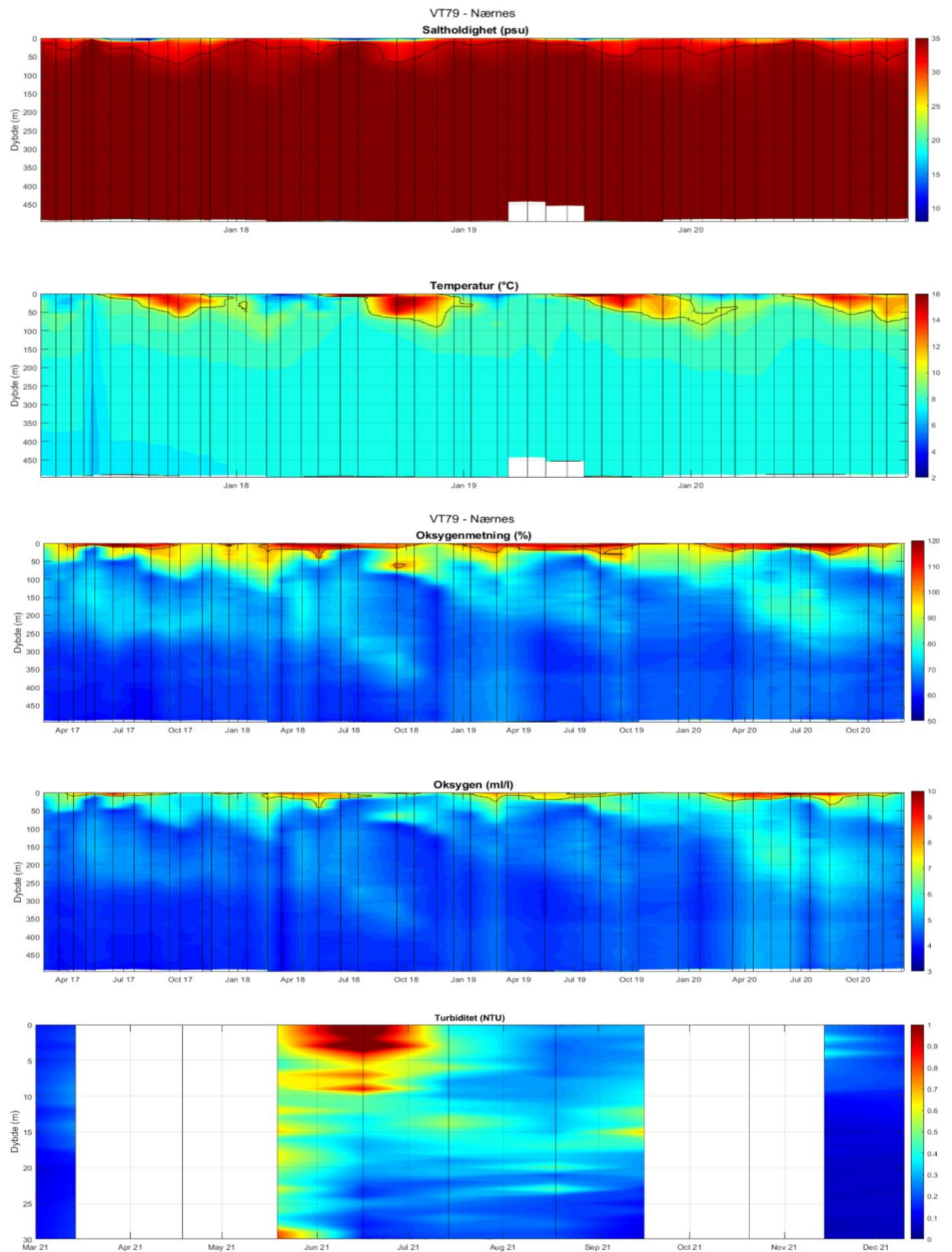
Figur 48. Data fra CTD-målinger på stasjon VT79 Nærnes. Øverst vises konturplott av saltholdighet med en fargeskala fra 10 til 35. Under saltholdighetsplottet vises konturplott av temperatur med en fargeskala fra 2 til 16 °C. Under temperaturplottet vises et konturplott av oksygenmetningen med en fargeskala fra 50 til 120%. Videre vises oksygenkonsentrasjonen med en fargeskala fra 3 til 10 ml/L. Nederst vises turbiditet fra 2021 for de øvre 30 meterne med en fargeskala fra 0 til 1 FNU. Sorte streker indikerer dato for når observasjonene ble gjort. Hvite felt indikerer manglende data.
