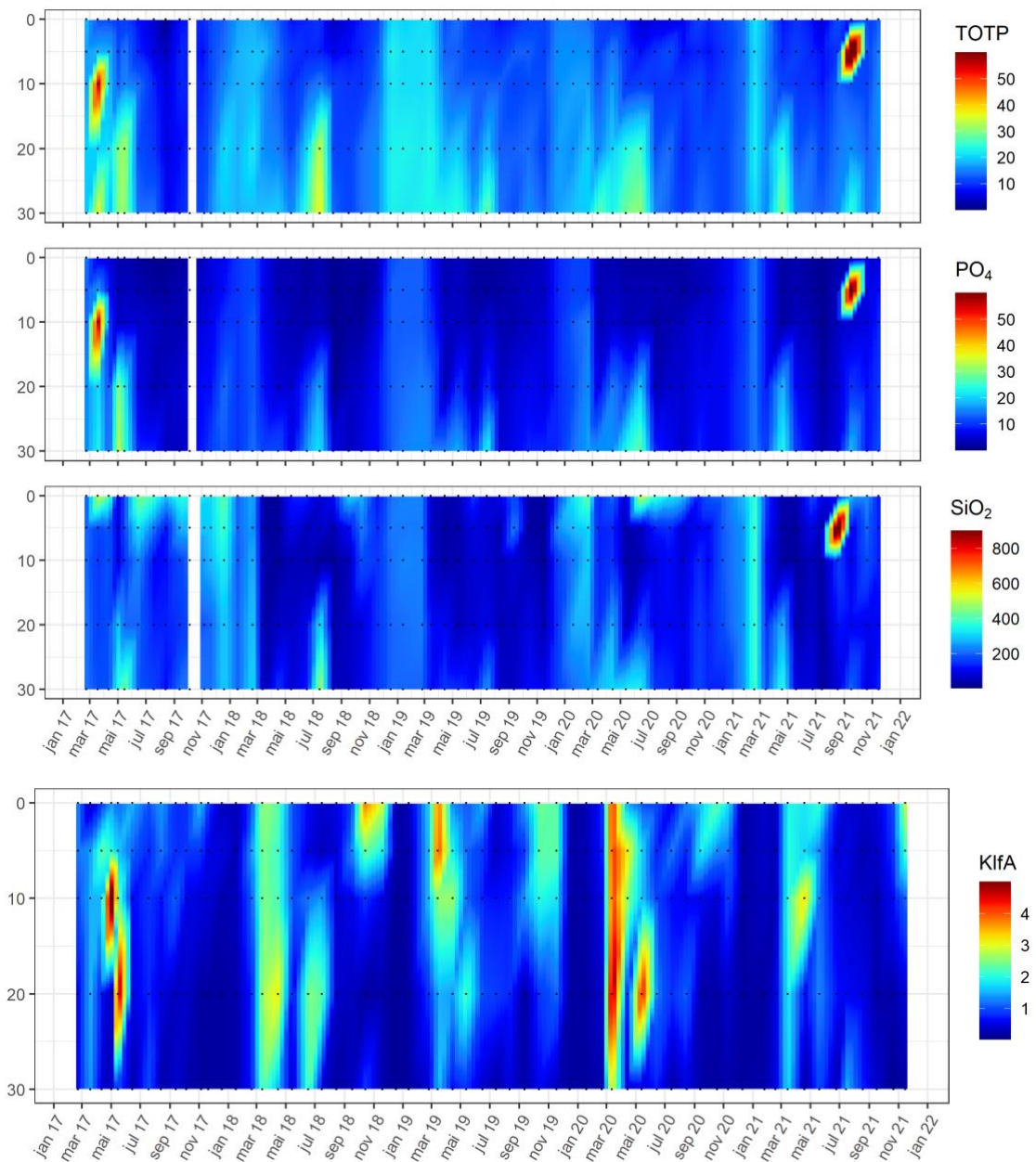
Figur 58. Næringssalter og klorofyll a som funksjon av tid og dyp for stasjon VT16 Kyrkjebø i perioden 2017 til 2021. Næringssalter for alle dyp mangler for oktober 2017 og SiO 2 mangler for november 2017. For nitrat mangler det målinger fra mai 2018 og juli 2018. Dette er rapportert som avvik tidligere. De svarte sirklene er prøvetidspunkt og prøvetakningsdyp.
