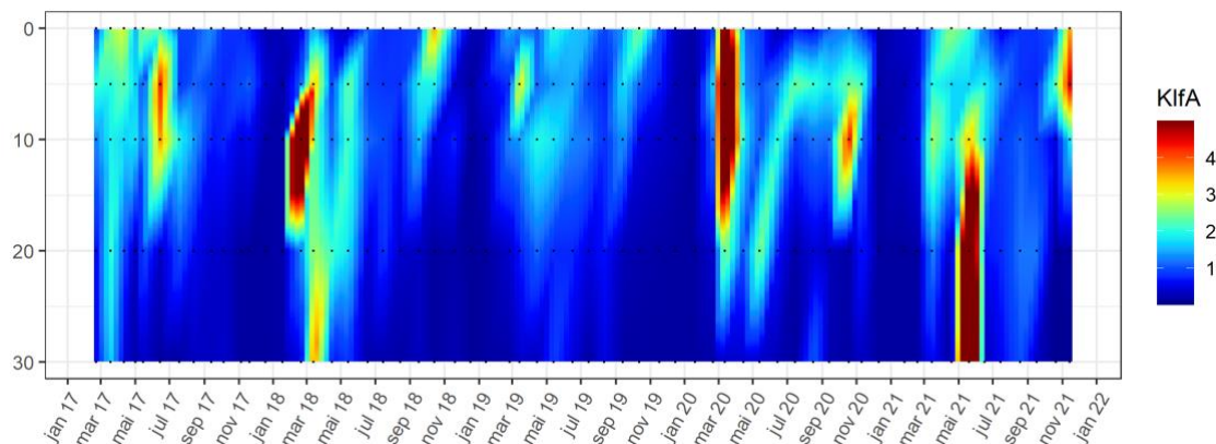
Figur 59. Næringssalter og klorofyll a som funksjon av tid og dyp for stasjon VT79 Nærnes i perioden 2017 til 2021. Næringssalter for alle dyp mangler for oktober 2017 og SiO 2 mangler for november 2017. For nitrat mangler det målinger fra mai 2018 og juli 2018. Dette er rapportert som avvik tidligere. De svarte sirkelene er prøvetidspunkt og prøvetakningsdyp.
