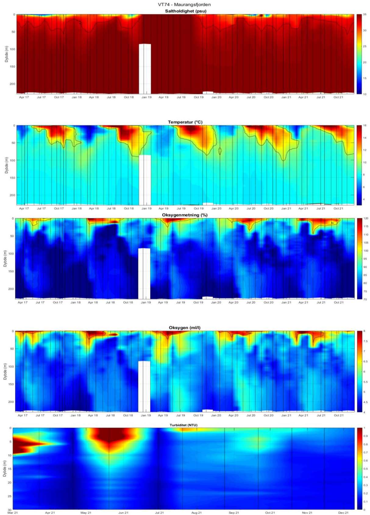
Figur 50. Data fra CTD-målinger på stasjon VT74 Maurangersfjorden. Øverst vises konturplott av saltholdighet med en fargeskala fra 10 til 35. Under saltholdighetsplottet vises konturplott av temperatur med en fargeskala fra 4 til 16 °C. Under temperaturplottet vises et konturplott av oksygenmetningen med en fargeskala fra 70 til 120%. Videre vises oksygenkonsentrasjonen med en fargeskala fra 4 til 8 ml/L. Nederst vises turbiditet fra 2021 for de øvre 30 meterne med en fargeskala fra 0 til 1 FNU. Sorte streker indikerer dato for når observasjonene ble gjort. Hvide felt indikerer manglende data.
