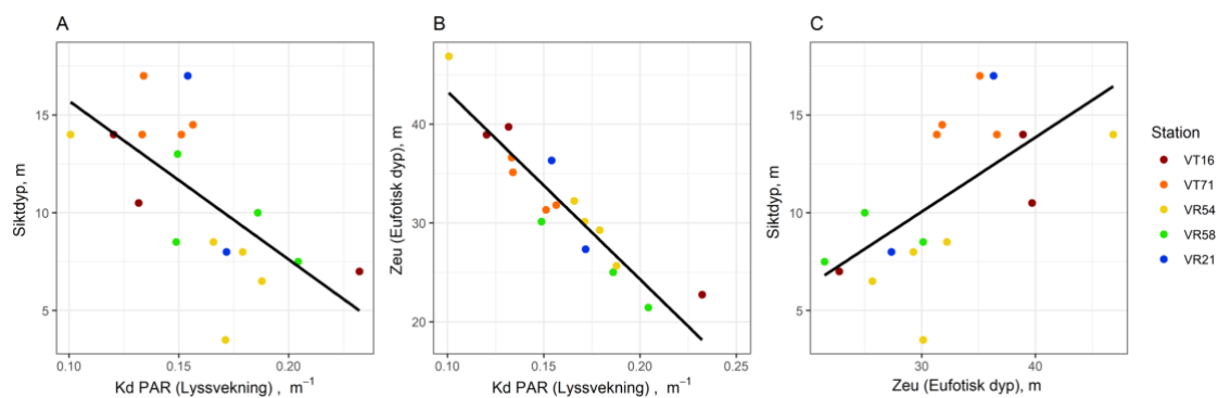
Figur 76. Siktdyp (m) i forhold til K_d PAR, lyssvekningskoeffisienten ( m^{-1} ) (A), Zeu, eufotisk dyp (m) i forhold til K_d PAR, lyssvekningskoeffisienten ( m^{-1} ) (B), siktdyp (m) i forhold til Zeu, eufotisk dyp (m) (C). Farger indikerer de ulike stasjonene fra syd til nord.
