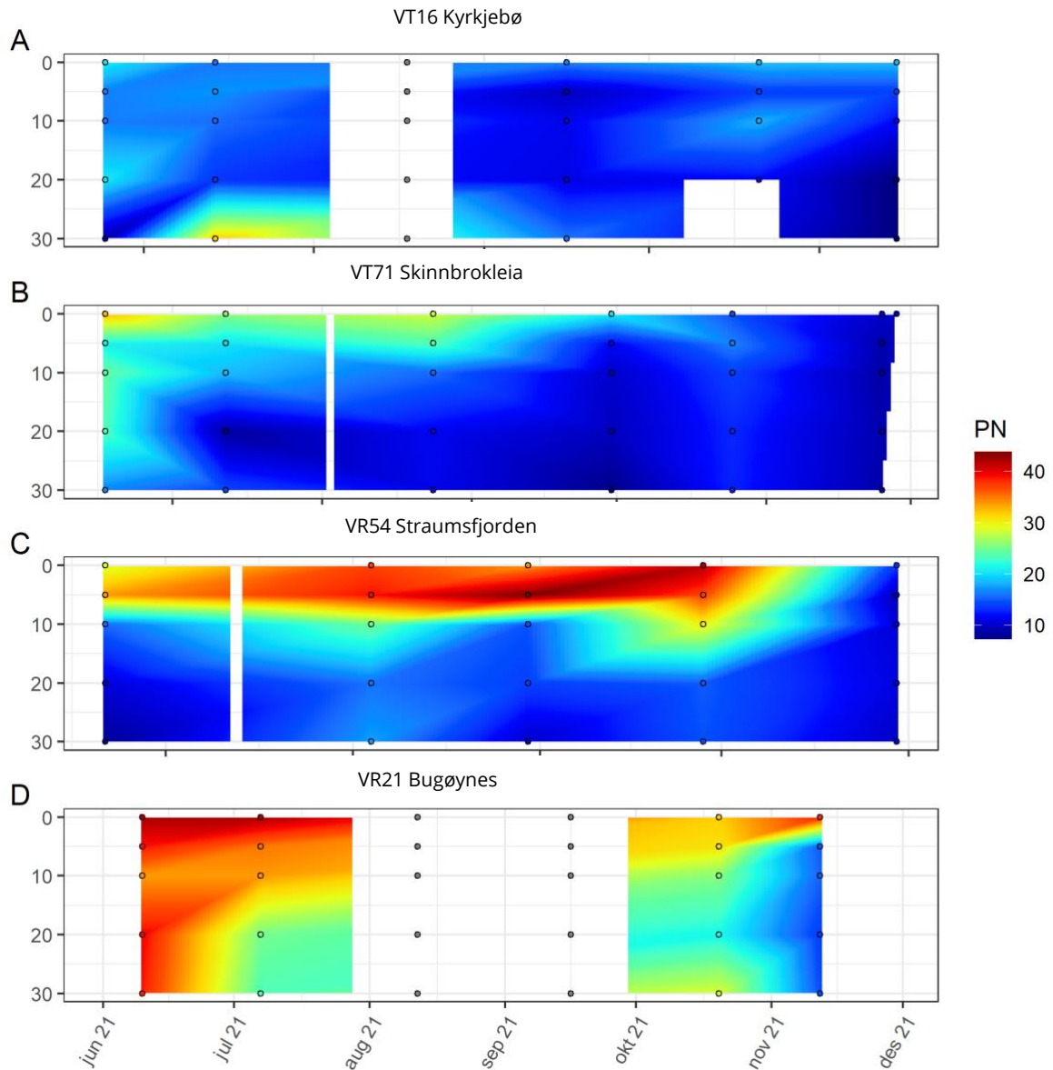
Figur 73. Partikulært nitrogen (PN) i 0-30 m dyp juni-november 2021 for klimastasjonene VT16 Kyrkjebø (A), VT71 Skinnbrokleia (B), VR54 Straumfjorden (C) og VR21 Bugøynes (D). Stasjon VR58 Ulsfjorden har ikke hatt målinger for denne parameteren i inneværende periode.
