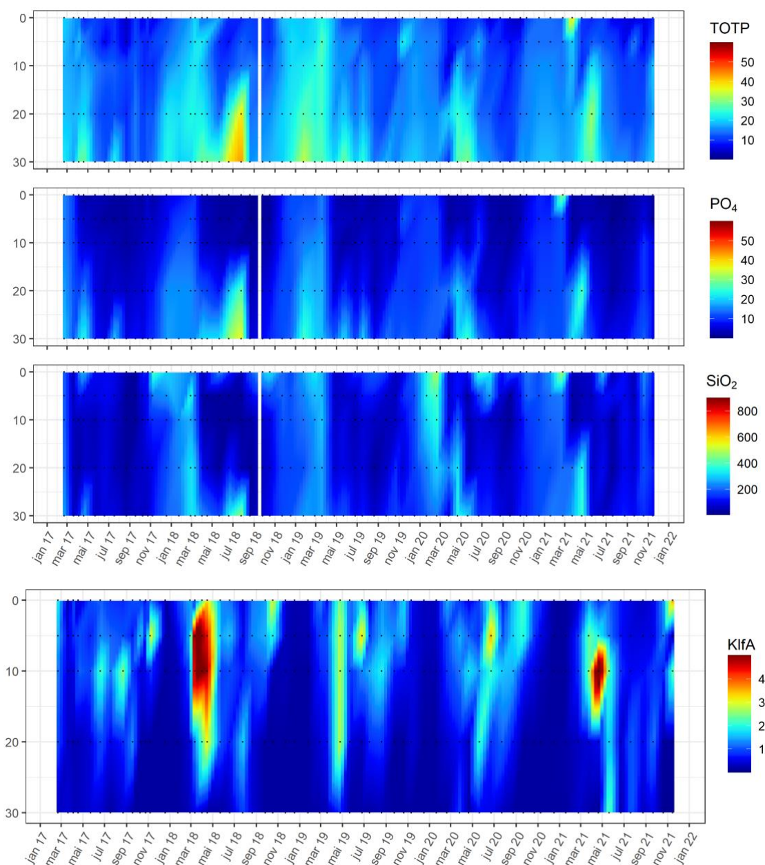
Figur 62. Næringssalter og klorofyll a som funksjon av tid og dyp for stasjon VT53 Tveiteneset i perioden 2017 til 2021. For september 2018 mangler det næringssalter for alle dyp, og dette er rapportert som avvik tidligere. Andre hvite felter er data som er fjernet under kvalitetskontroll. De svarte prikkene er prøvetidspunkt og prøvetakningsdyp.
